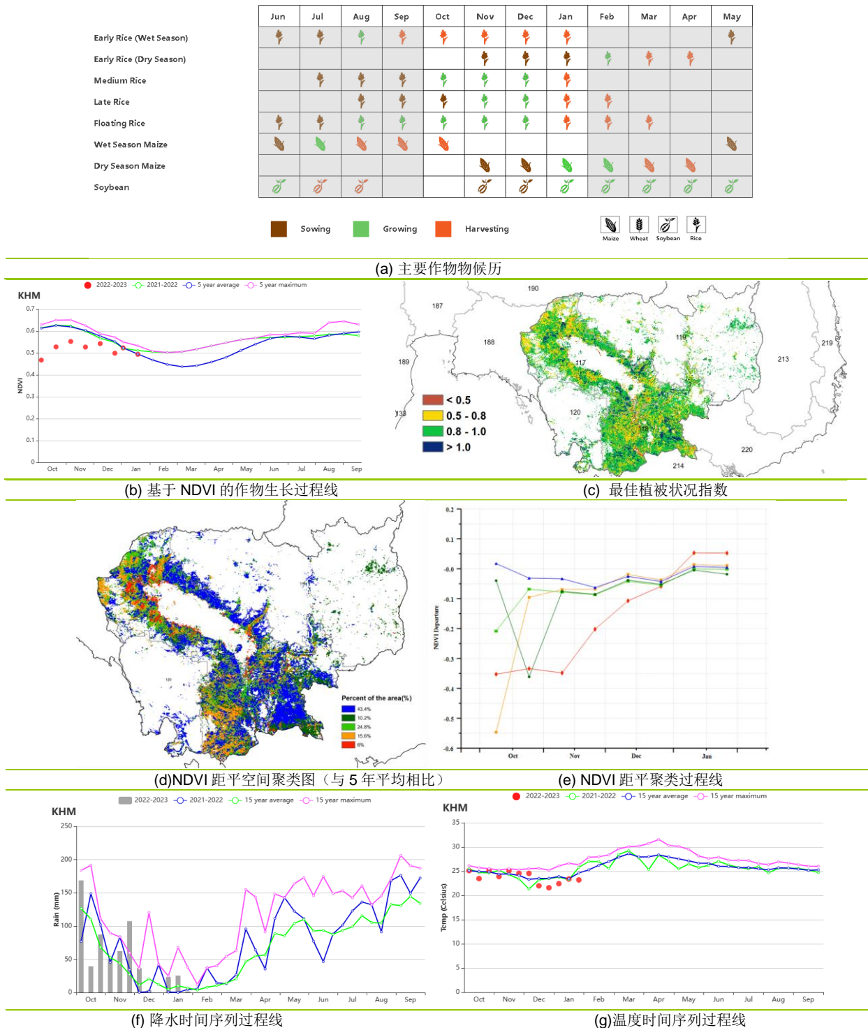
图 3.27 2022 年 10 月-2023 年 1 月柬埔寨作物长势
