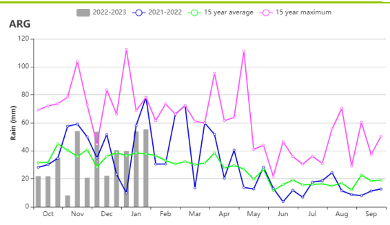
(g) 降水时间序列过程线 (阿根廷)
