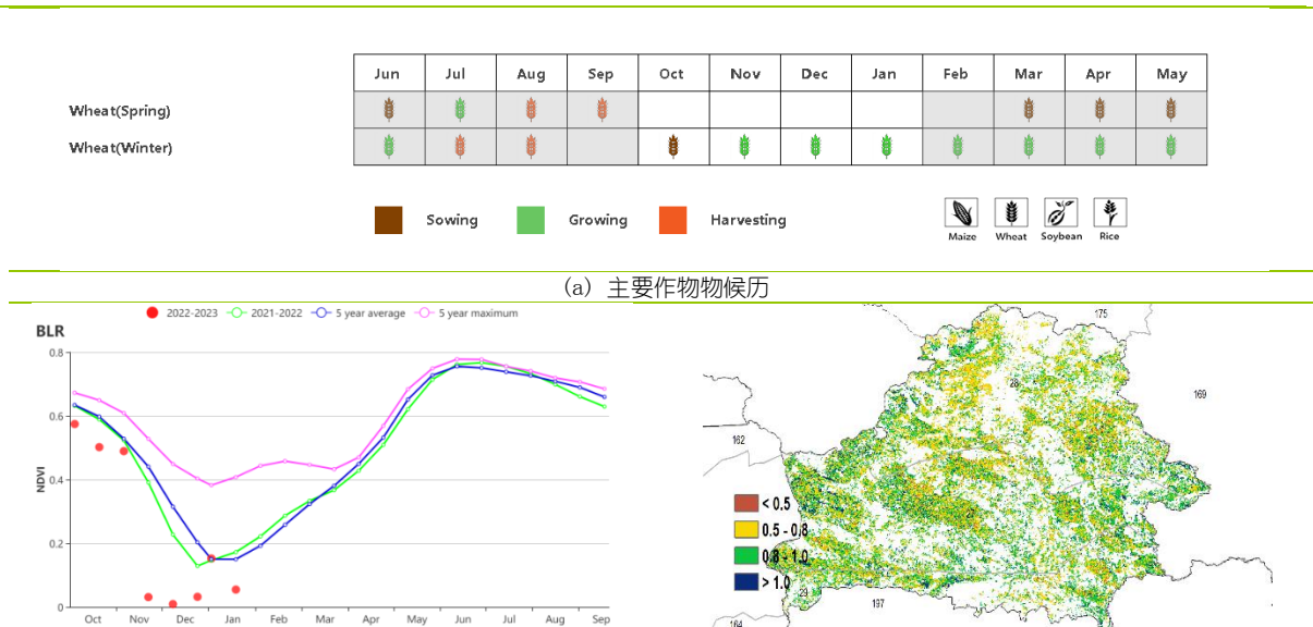
图 3.10 2022 年 10 月- 2023 年 1 月白俄罗斯作物长势
