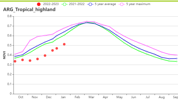
(f) 基于 NDVI 的作物生长过程线 (热带丘陵地区 阿根廷)
