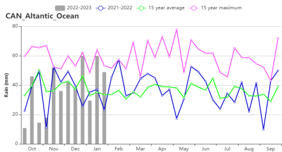
(h) 大西洋区降水时间曲线
