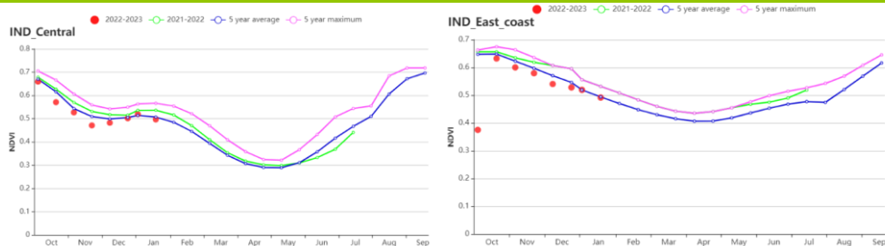
(h) 基于 NDVI 的作物生长过程线（德干高原（左）和东部沿海地区（右））
