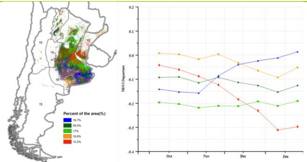
(i) NDVI 距平空间聚类图
