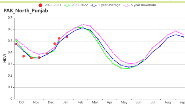
(h) 基于 NDVI 的作物生长过程线 (旁遮普北部)
