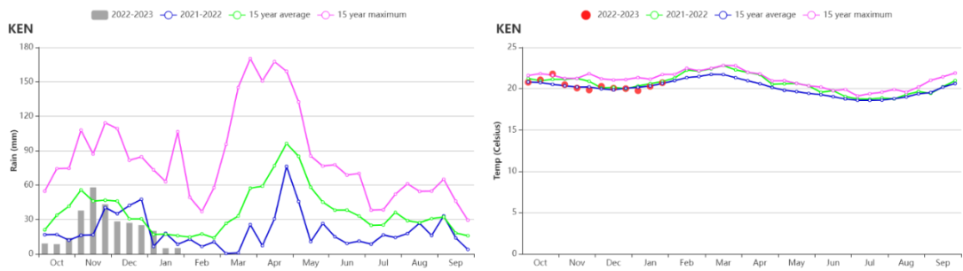
(f) 降水时间过程线
