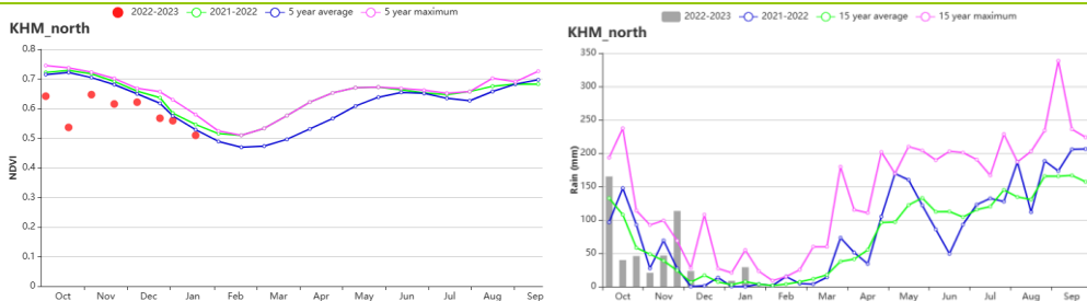
(j) 北部平原和东北区基于 NDVI 的作物生长过程线 (左) 和降水时间序列分布 (右)
